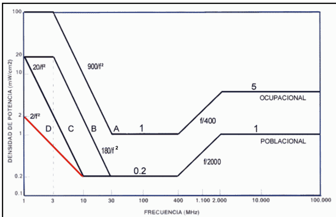
Gráfico IV: Valores límite para exposición de seres humanos a Radiofrecuencias y Microondas, establecidos por Resolución MS 202/1995 y Ratificados por resolución SeCom 530/2000 (Ambas en vigencia).
