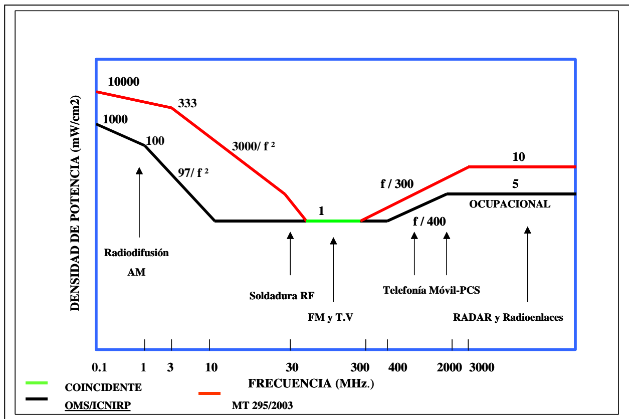
Gráfico comparativo. Resolución MT295/2003-Valores OMS/ICNIRP
