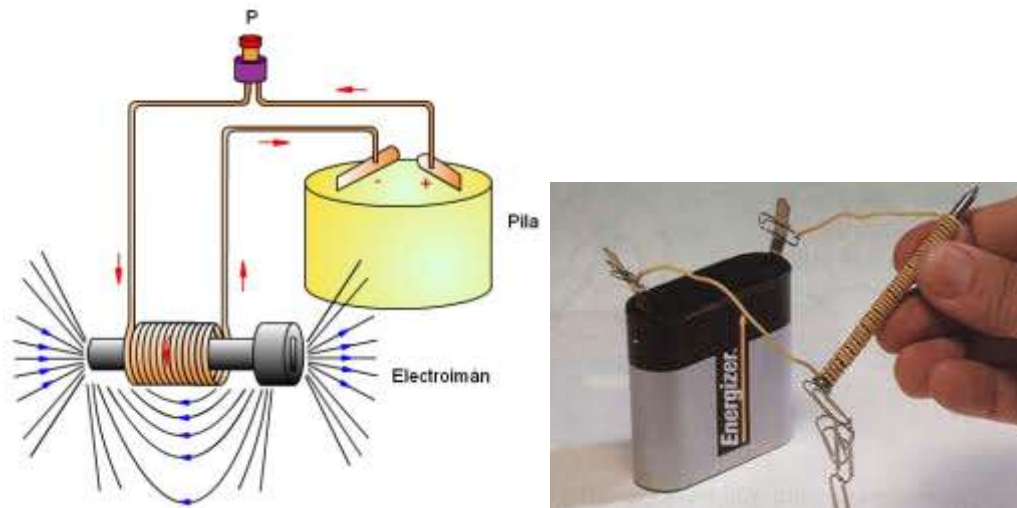
Figura 14: ejemplo de electroimán.
