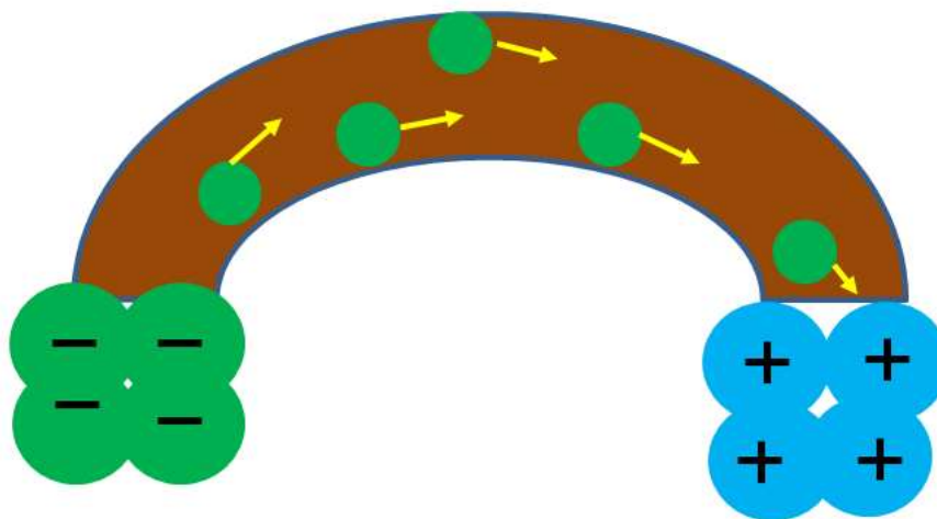
Figura 3: electrones libres en un "cable" de cobre, moviéndose ordenadamente por la fuerza de atracción.
