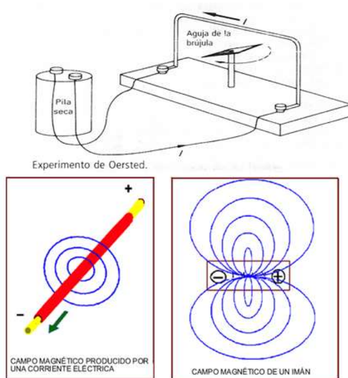
Figura 6: Experimento de Oersted, y formas del Campo Magnético alrededor de un conductor con corriente y de un imán.
