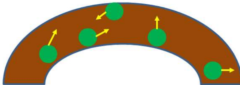
Figura 2: electrones libres en un "cable" de cobre, moviéndose aleatoriamente.
