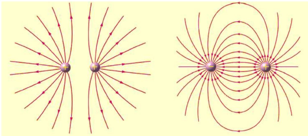
Figura 12: Líneas de Campo Eléctrico para un sistema elemental de dos cargas, en un caso iguales, en el otro opuestas.
