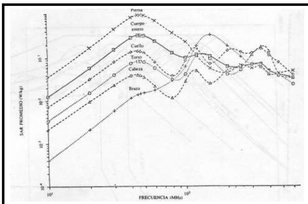
Grafico III: Variación de la tasa SAR promedio en función de la frecuencia y la zona del cuerpo radiada.
