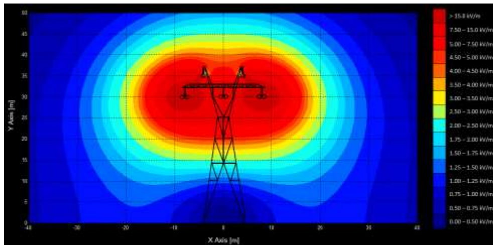
Figura 16: Distribución de Campo Eléctrico en una línea de alta tensión de 50Hz
