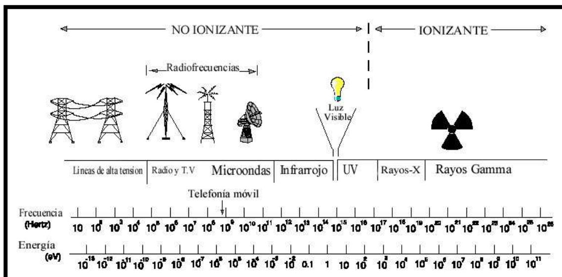
Gráfico II: Espectro electromagnético: algunos servicios fundamentales, sus energías y frecuencias. (Fuente FCC)
