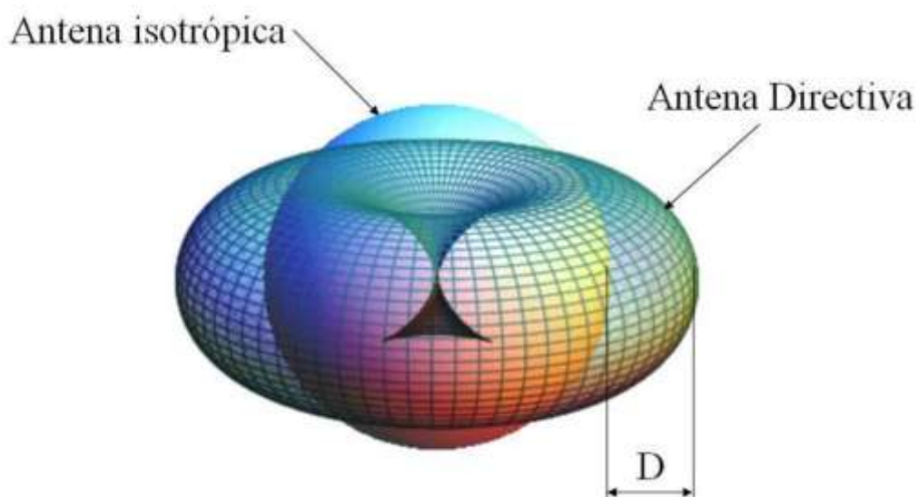
Figura 20: Diferencia entre un Diagrama isotrópico y un diagrama más directivo
