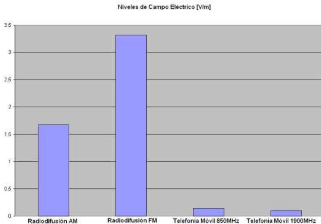
Gráfico VII: Niveles de Campo por Servicio, para la Ciudad de Buenos Aires (horario laboral)
