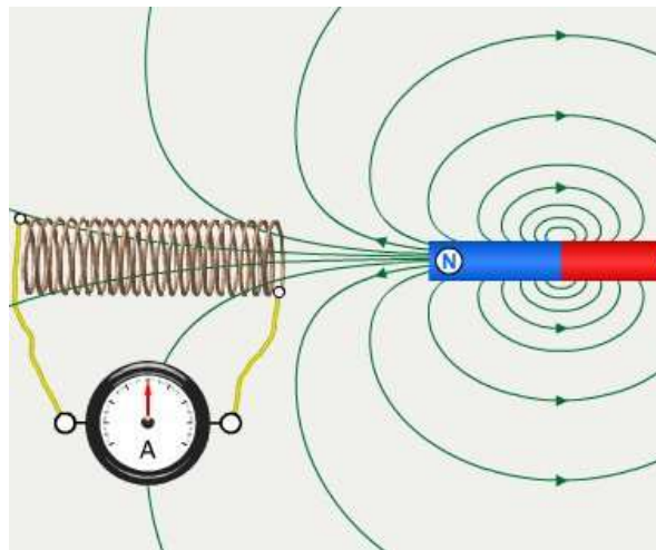
Figura 7: Representación esquemática del experimento de Faraday
