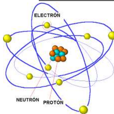
Figura 1: el átomo y sus partículas.
