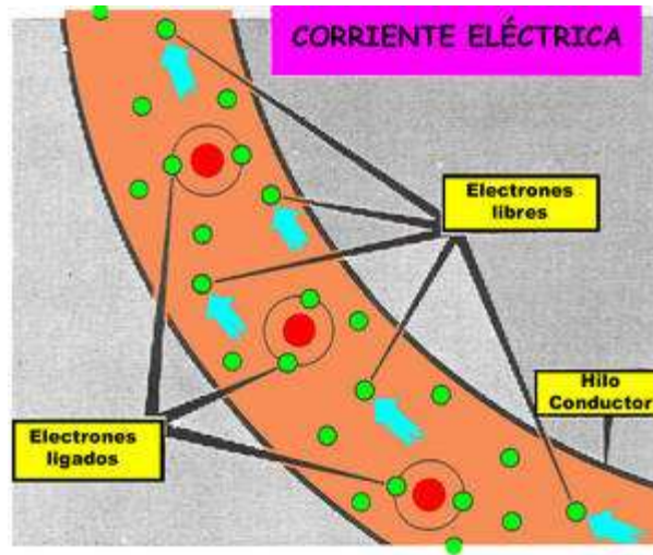
Figura 5: Corriente Eléctrica: movimiento ordenado de electrones libres por un conductor.
