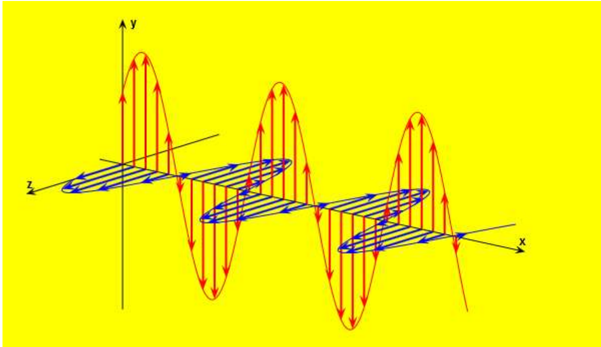
Figura 17: Onda Electromagnética. Campo Eléctrico en rojo y Campo Magnético en azul
