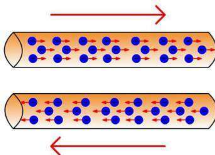
Figura 8: Movimiento de electrones para una Corriente Alterna
