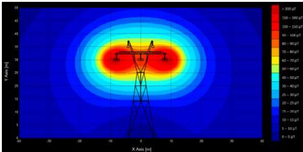
Figura 15: Distribución de Campo Magnético en una línea de alta tensión de 50Hz
